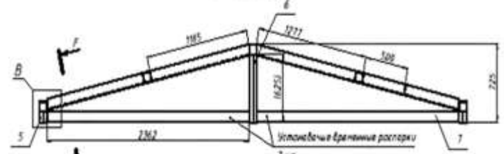
A-A (1:15)
